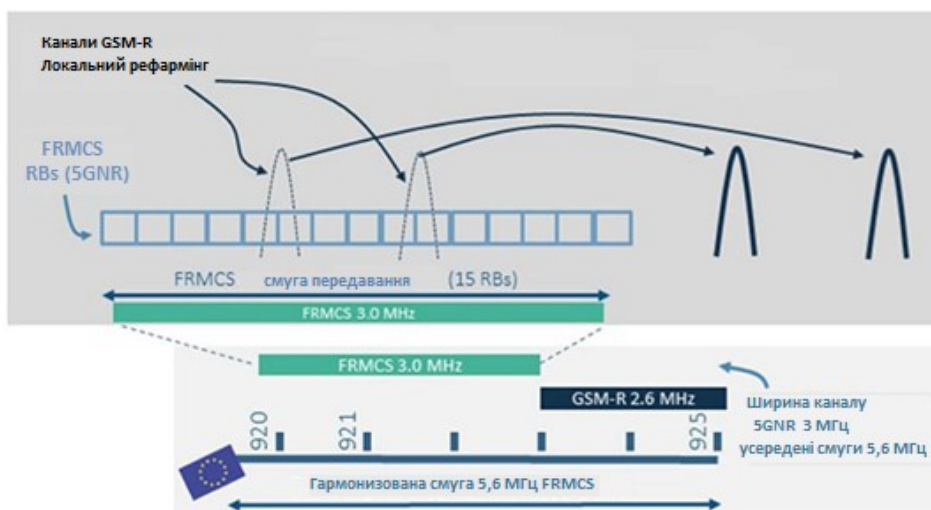
Рис. 3. Трансформація спектру 900 МГц для FRMCS [8]
